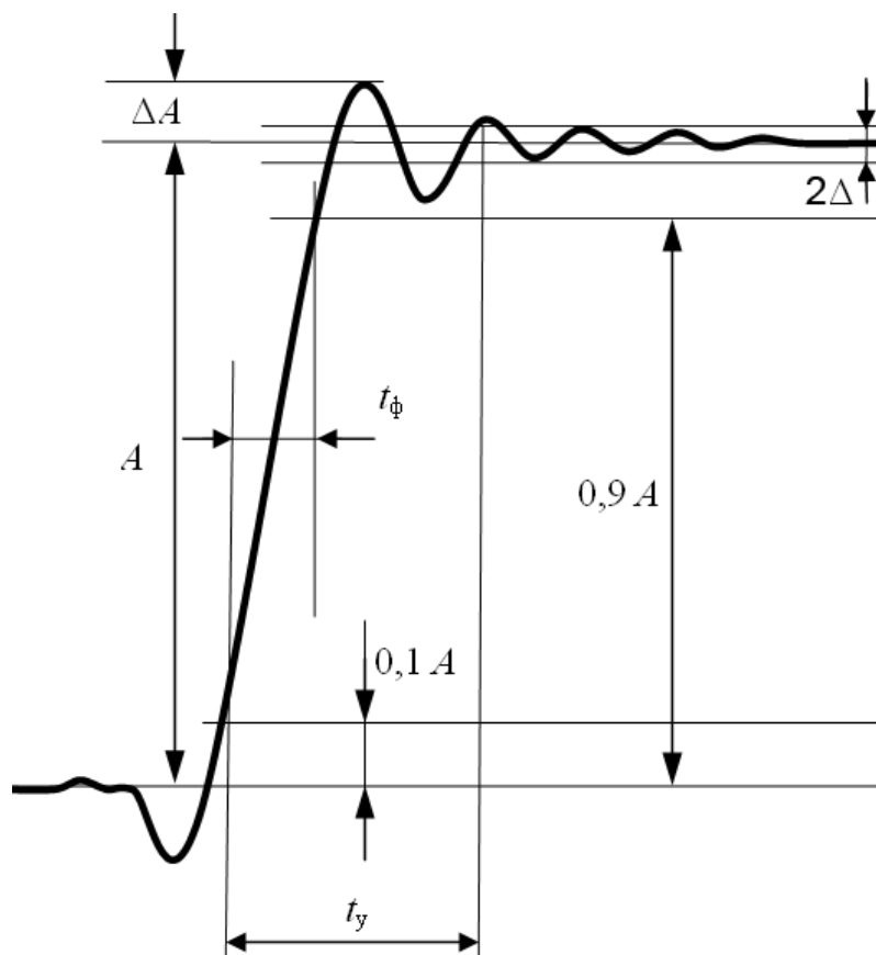
Рисунок 7.4 - Переходная характеристика (ПХ) и ее параметры:
