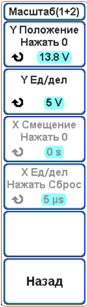
Рисунок 6.12 – Экранное меню «Масштаб (1+2)»
