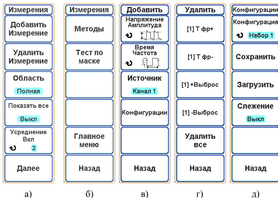
Рисунок 6.25 – Экранное меню а) «Измерения» (основное); б) «Измерения» (дополнительное); в) «Добавить», г) «Удалить» д) Конфигурации
