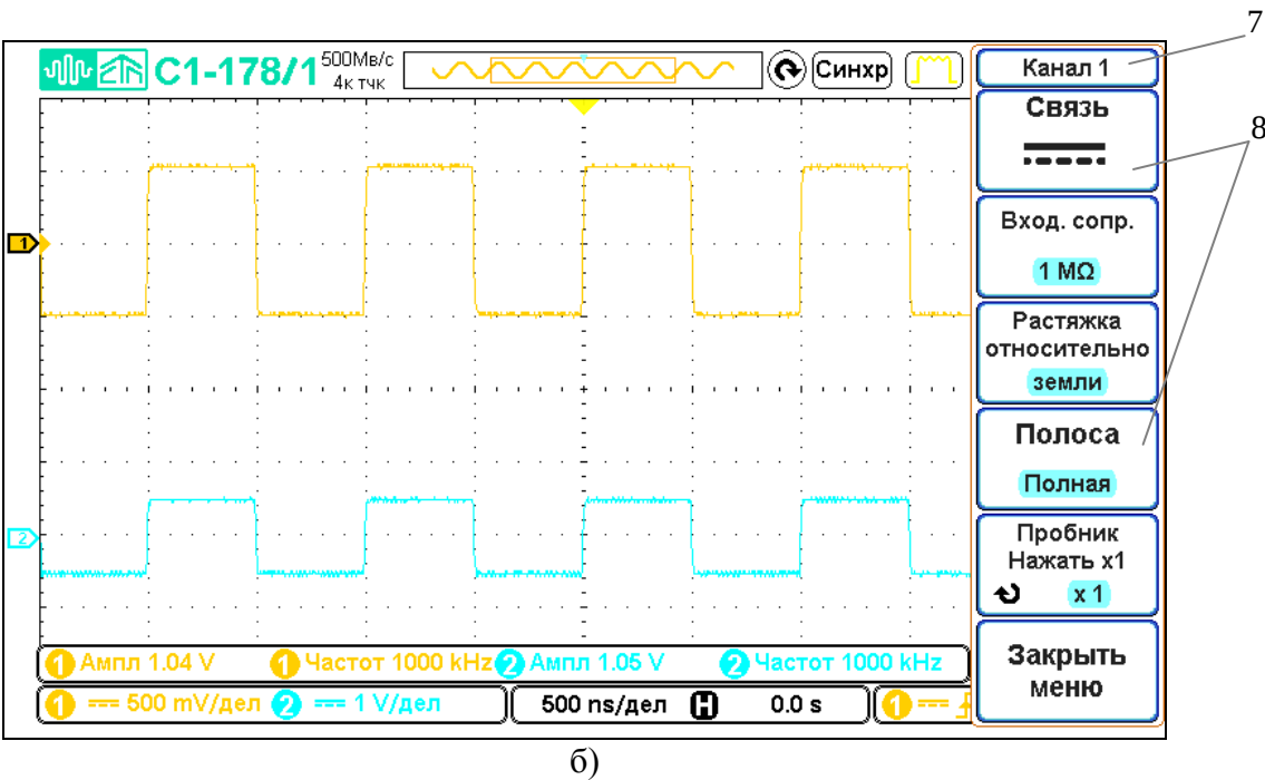
Рисунок 6.3 – Интерпретация показаний на экране осциллографа
