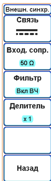
Рисунок 6.23 – Экранное меню «Внешняя синхронизация»
