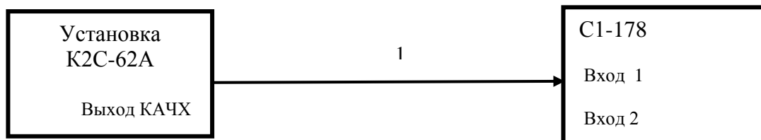
Рисунок 7.2 – Схема соединения приборов для проверки коэффициентов развертки
