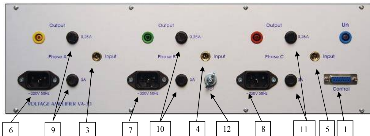
Рисунок 1.13 - Вид лицевой панели усилителя напряжения "УН-3.1"
