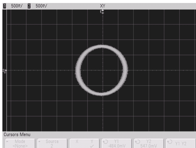
Рис. 21 Фазовый сдвиг между сигналами равен 90°
