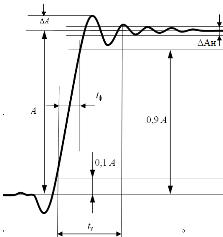
Рисунок 7.4 - Переходная характеристика (ПХ) и ее параметры:
