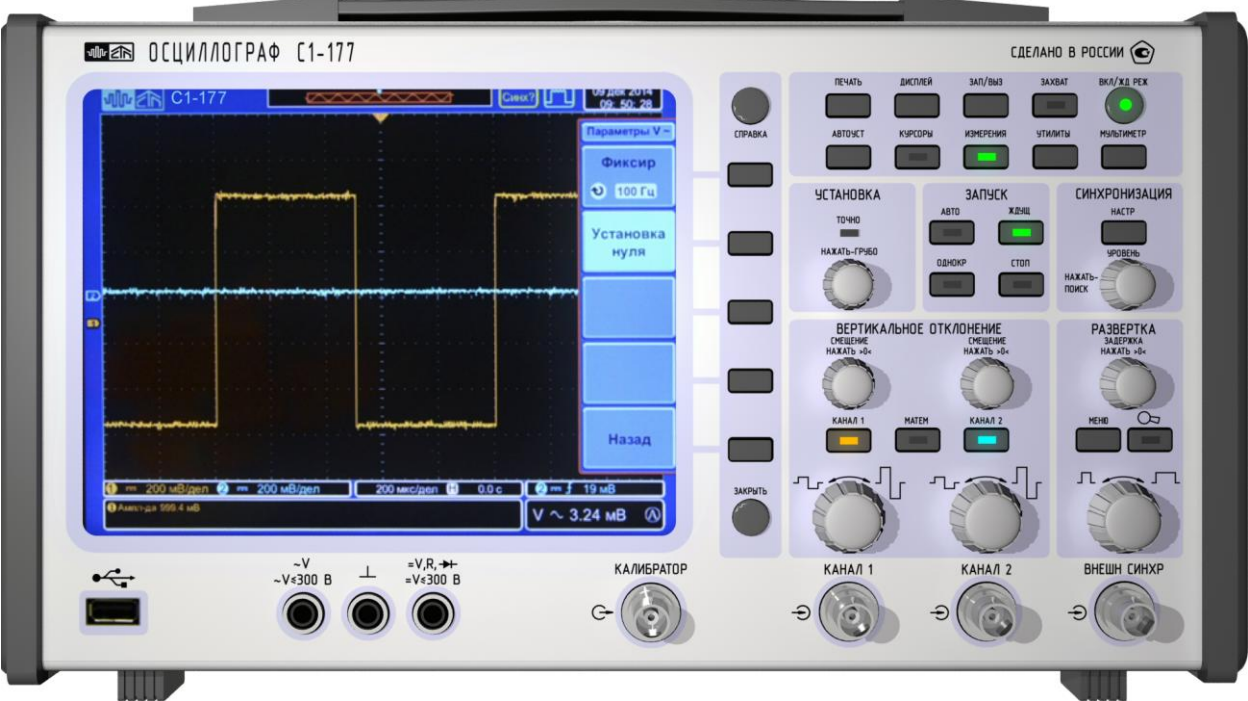
Рисунок 1 – Внешний вид осциллографа С1-177
