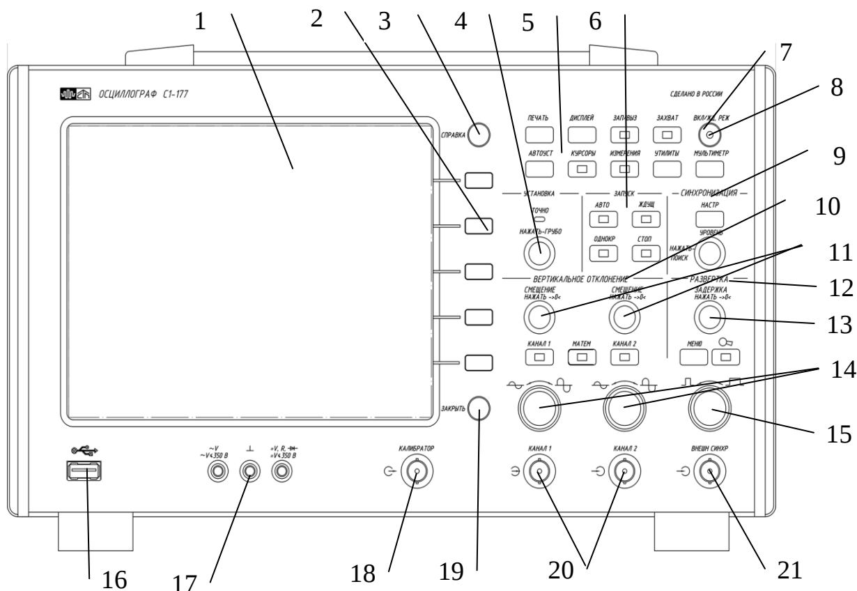
Рисунок 6.1 – Передняя панель осциллографа
