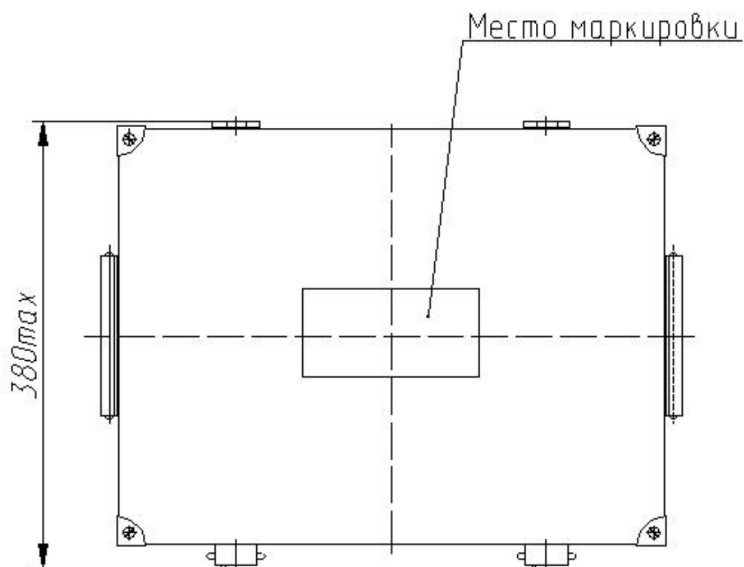
Рисунок 4.2 – Габаритные размеры ящика укладочно-транспортного, мм
