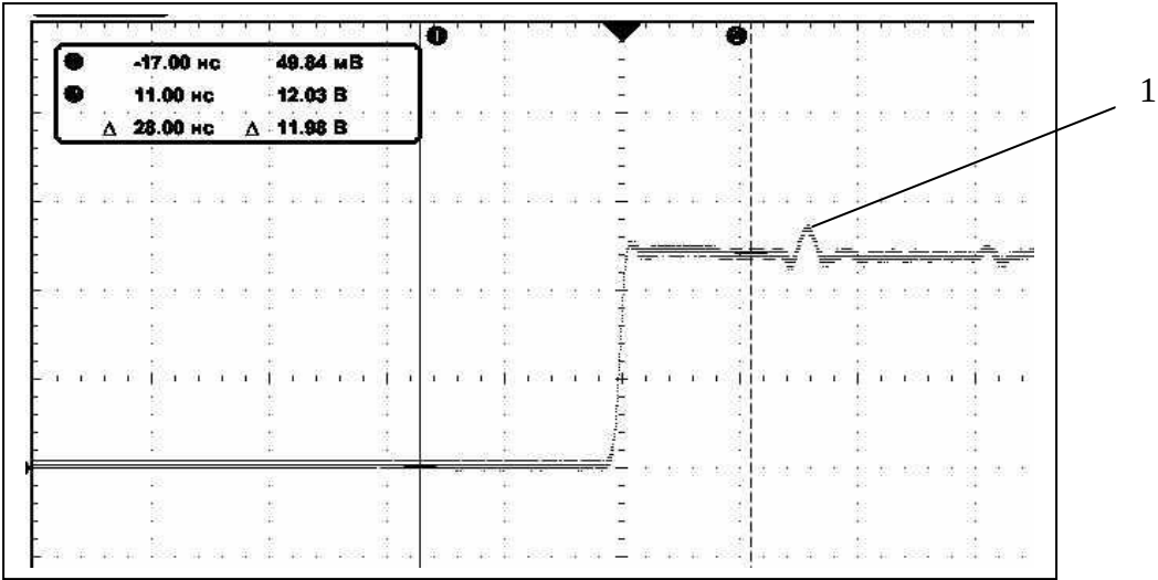
Рисунок 7.4.1 – Исключение неравномерности вершины (1) сигнала калибратора K2C-62A
