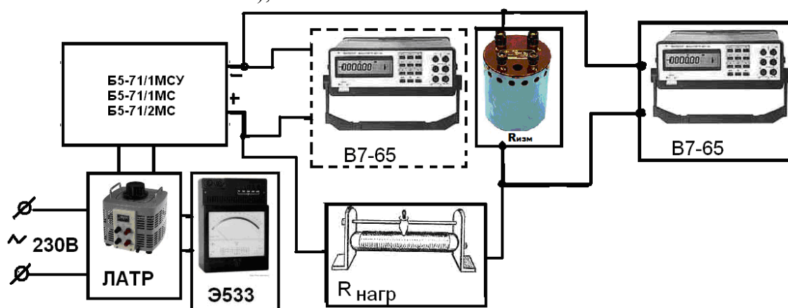
Рисунок 4 – Схема измерения нестабильности выходного тока от изменения напряжения питающей сети в режиме стабилизации тока
